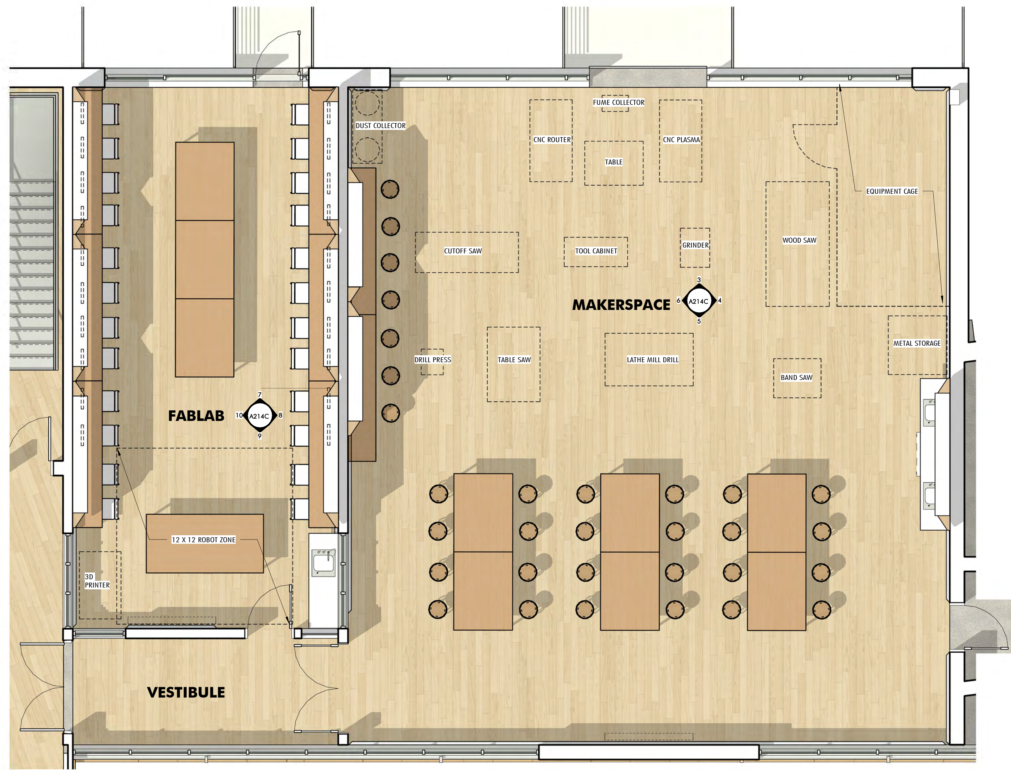
PLAN - FABLAB AND MAKERSPACE
